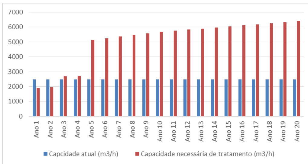
Figura 30. Variação da capacidade de tratamento de esgotos necessária no município de Natal em função das metas estabelecidas pelo Cenário 1.
